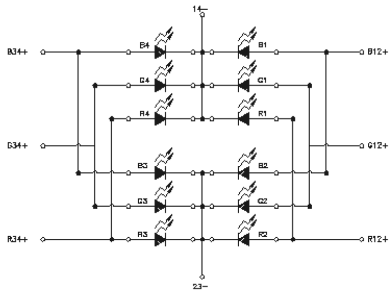
Polarity
